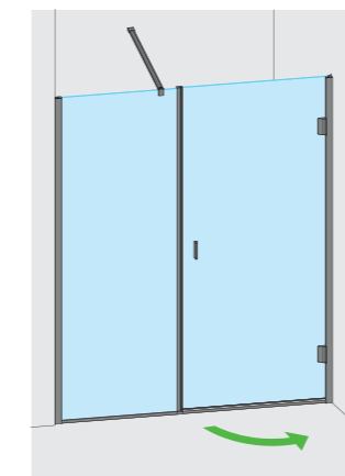
MOD. SINISTRO CON POMOLO A SINISTRA, LATO FISSO A SINISTRA
