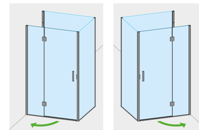
MOD. DESTRO CON MANIGLIA A DESTRA 2 LATI FISSI A DESTRA
